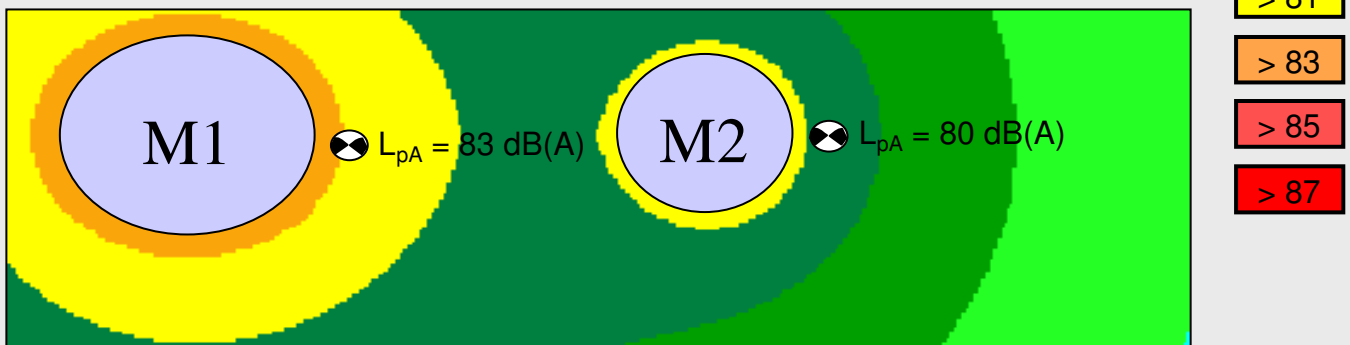
Abb. 4: Lärmkarte Mischerhalle, Mischer M1 zusätzlich lärmgemindert um 5 dB(A)
