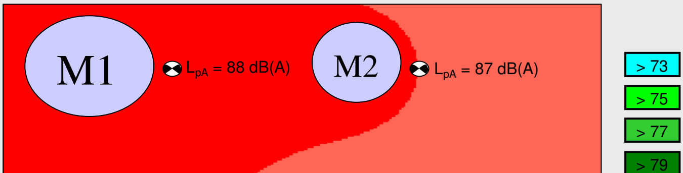
Abb. 3: Lärmkarte Mischerhalle mit schallabsorbierender Hallendecke
