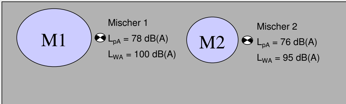
Abb. 1: Mischerhallengrundriss (L=30m, B=10m, H=4m) mit normgerechten Geräuschangaben des Herstellers
