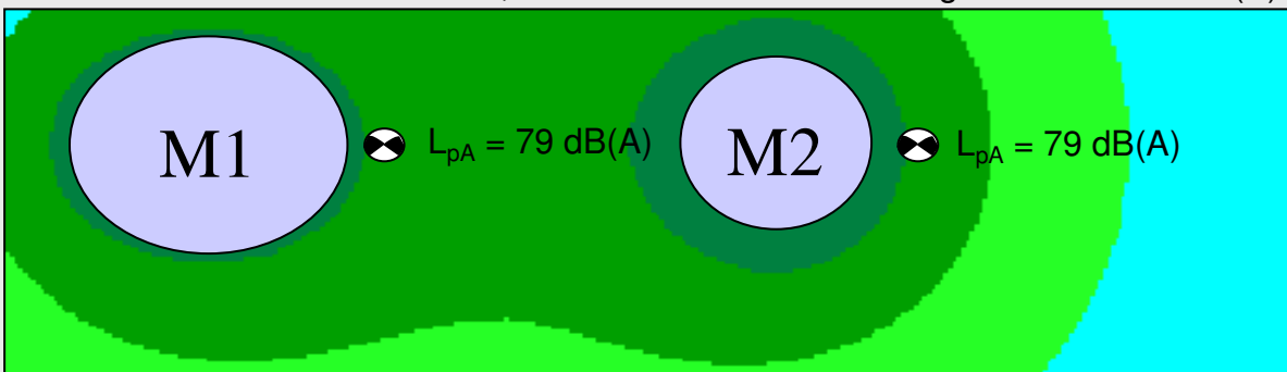
Abb. 4: Lärmkarte Mischerhalle, Mischer M1 zusätzlich lärmgemindert um 5 dB(A)
